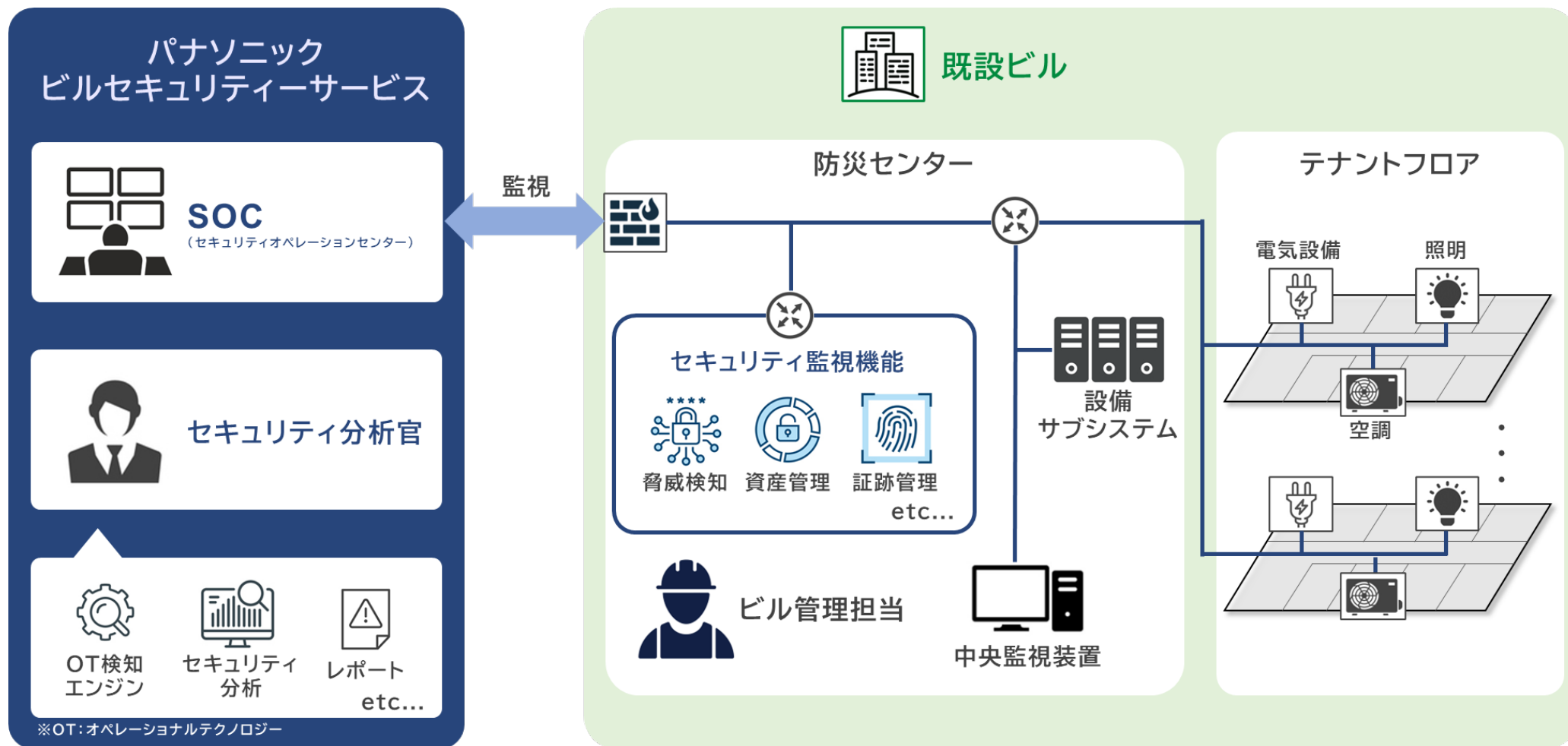
ビル向けサイバーセキュリティ監視システムの構成図
